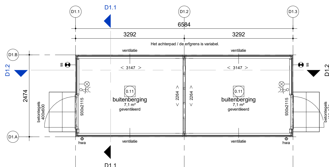
Begane grond
