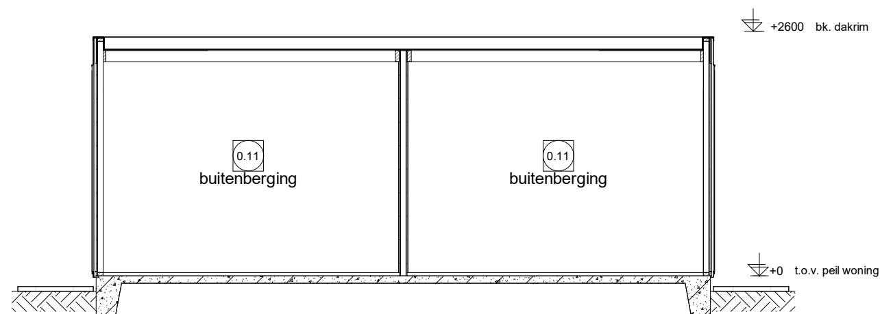
Doorsnede D1.2
