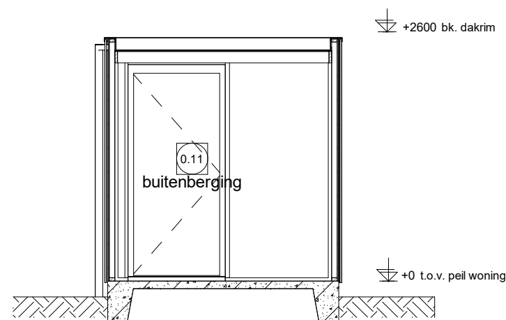
Doorsnede D1.1
