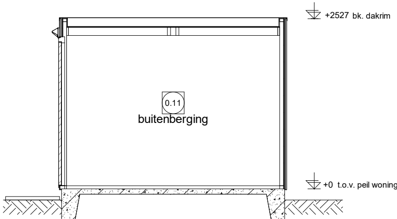
Doorsnede F1.2
