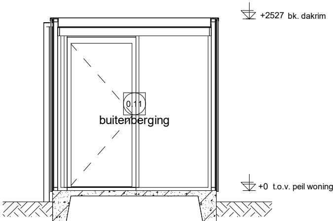
Doorsnede F1.1
