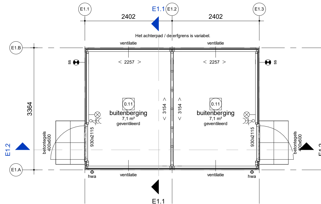
Begane grond
