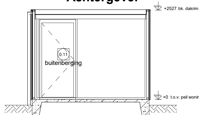
Doorsnede E1.1
