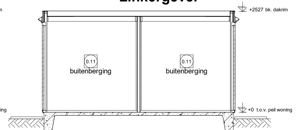
Doorsnede E1.2
