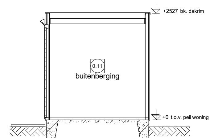
Doorsnede F2.2
