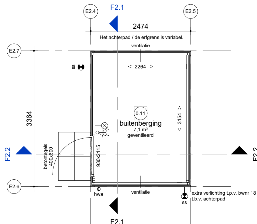
Begane grond
