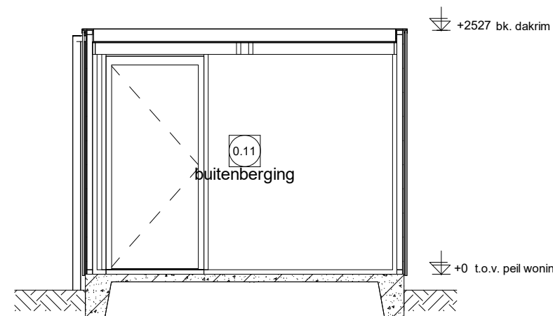
Doorsnede F2.1
