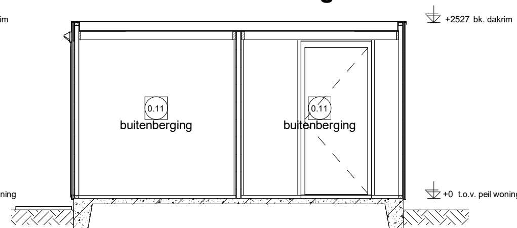
Doorsnede E3.2
