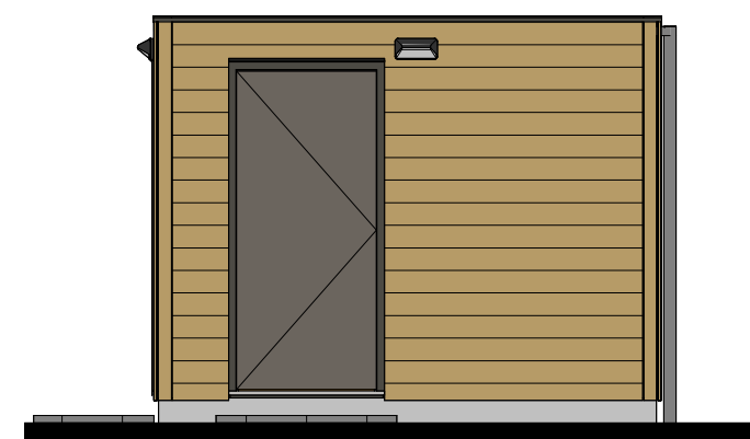
Linkergevel
